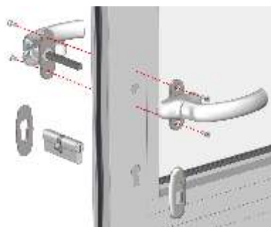
Poignées avec rosaces et canon de sécurité
