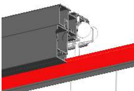
Joint d'étanchéité EPDM sur linteau
