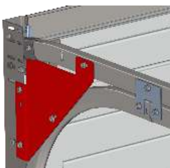
Plaqué renfort sur courbes
