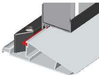
Seuil bas drainé en aluminium avec évacuation d'eau
