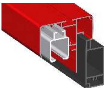
Précadre avec profil de rail monobloc
