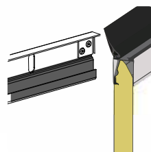
Joint haut sur traverse + joint à lèvre sur panneau haut
