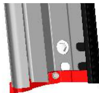
Système anti-corrosion pour pied de rail (en option)
