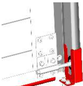
Sabot anti-effraction Sécurise le galet inférieur Fixé sur le rail vertical et au sol
