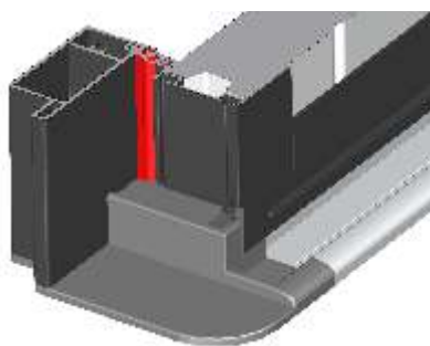
Joint d'étanchéité tubulaire EPDM côté ouverture
