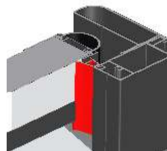
Joint tubulaire à lèvre EPDM côté fermeture
