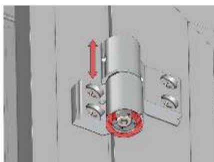
Réglage hauteur et profondeur
